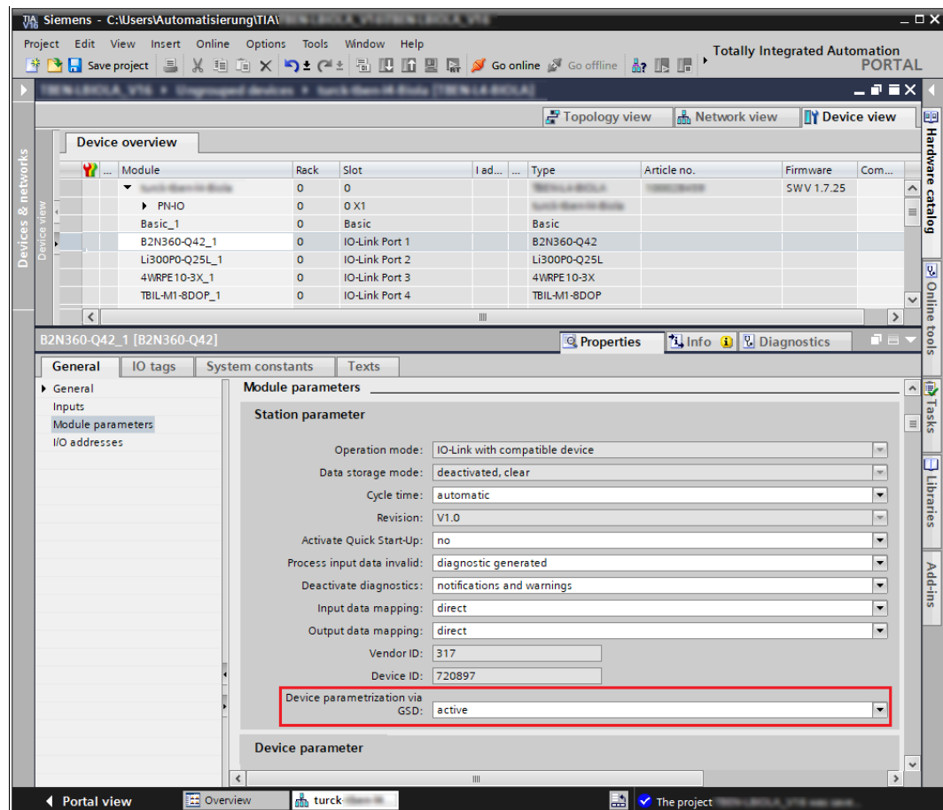
Fig. 72: Example: TIA Portal, "Device parameterization via GSD" parameter
