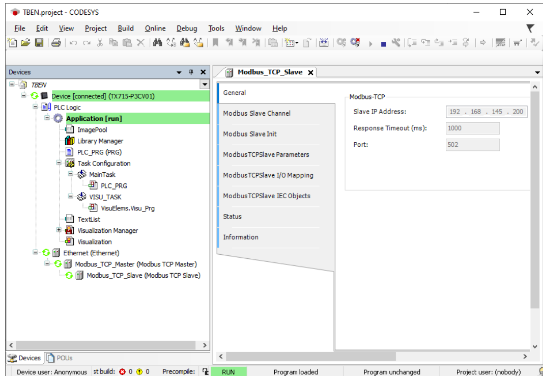
Fig. 44: Modbus TCP communication
