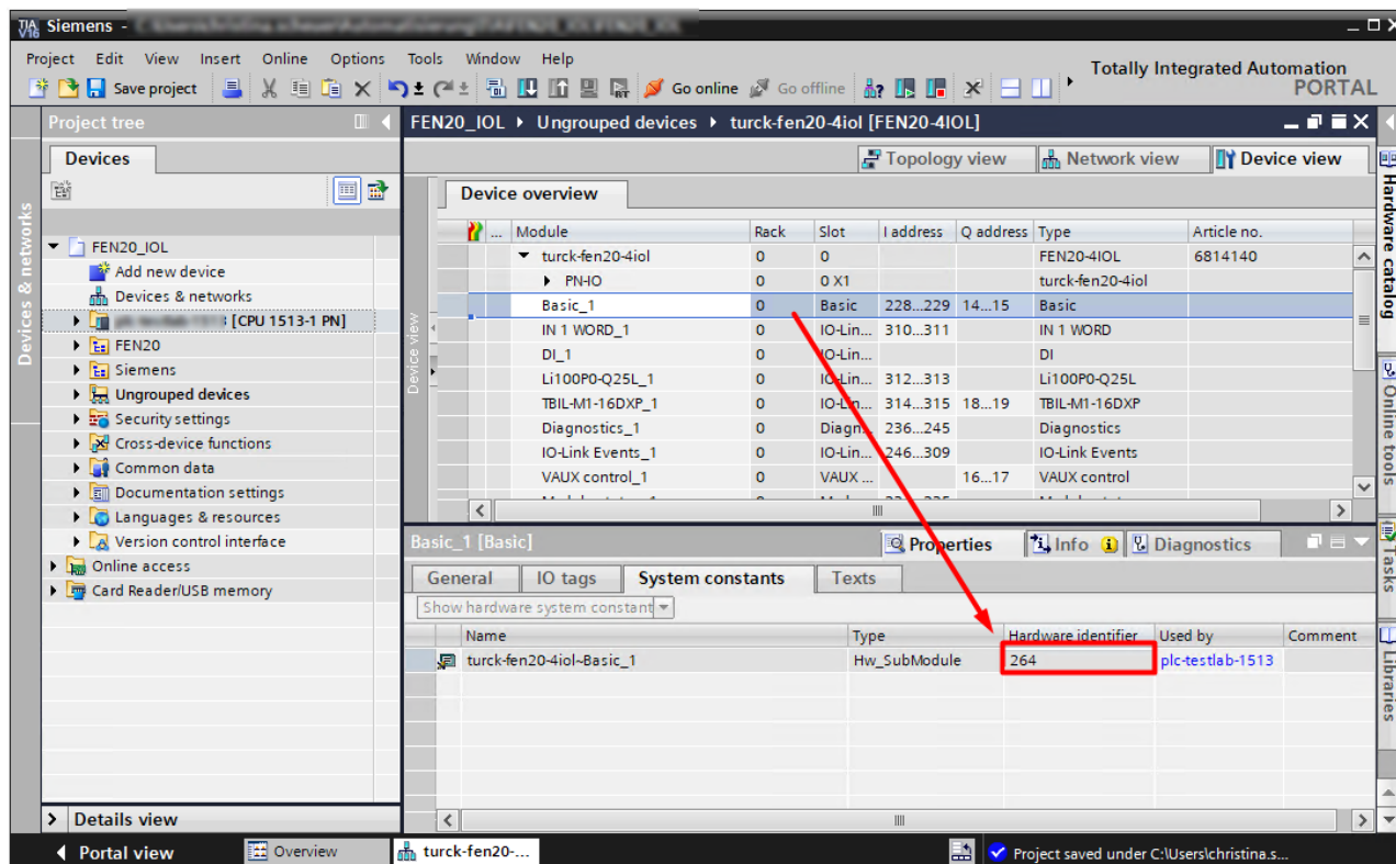
Fig. 27: HW identifier: „Basic“ slot (here: FEN20-4IOL)
