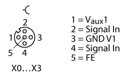
M12 × 1 Input
