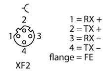
M12 × 1 Input
