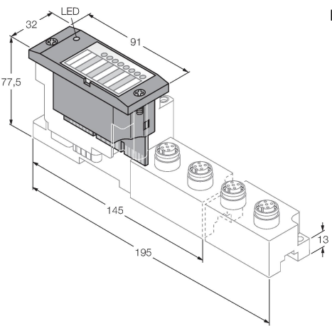
BL67-4IOL
